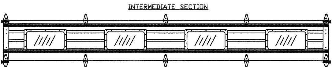
OPTIONAL GLAZED SECTION W/ 24' X 12' WINDOWS N.T.S.
