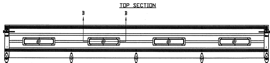
OPTIONAL GLAZED SECTION W/ 24' X 6' WINDOWS N.T.S.
