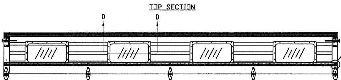
OPTIONAL GLAZED SECTION W/ 24' X 12' WINDOWS N.T.S.
