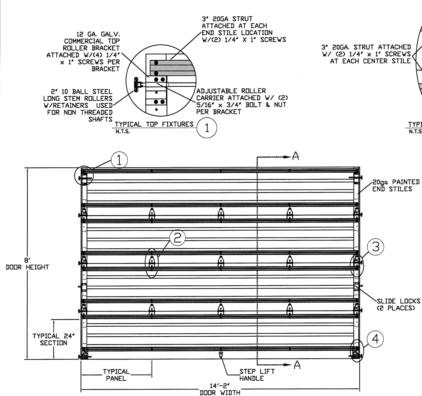
DOOR INTERIOR ELEVATION N.T.S.
