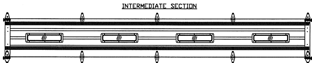
OPTIONAL GLAZED SECTION W/ 24' X 6' WINDOWS N.T.S.
